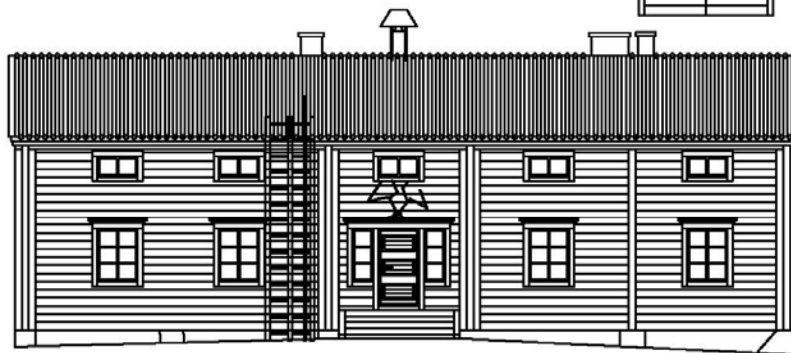
JULKISIVU ETUPIHALLE JUHONTALO
